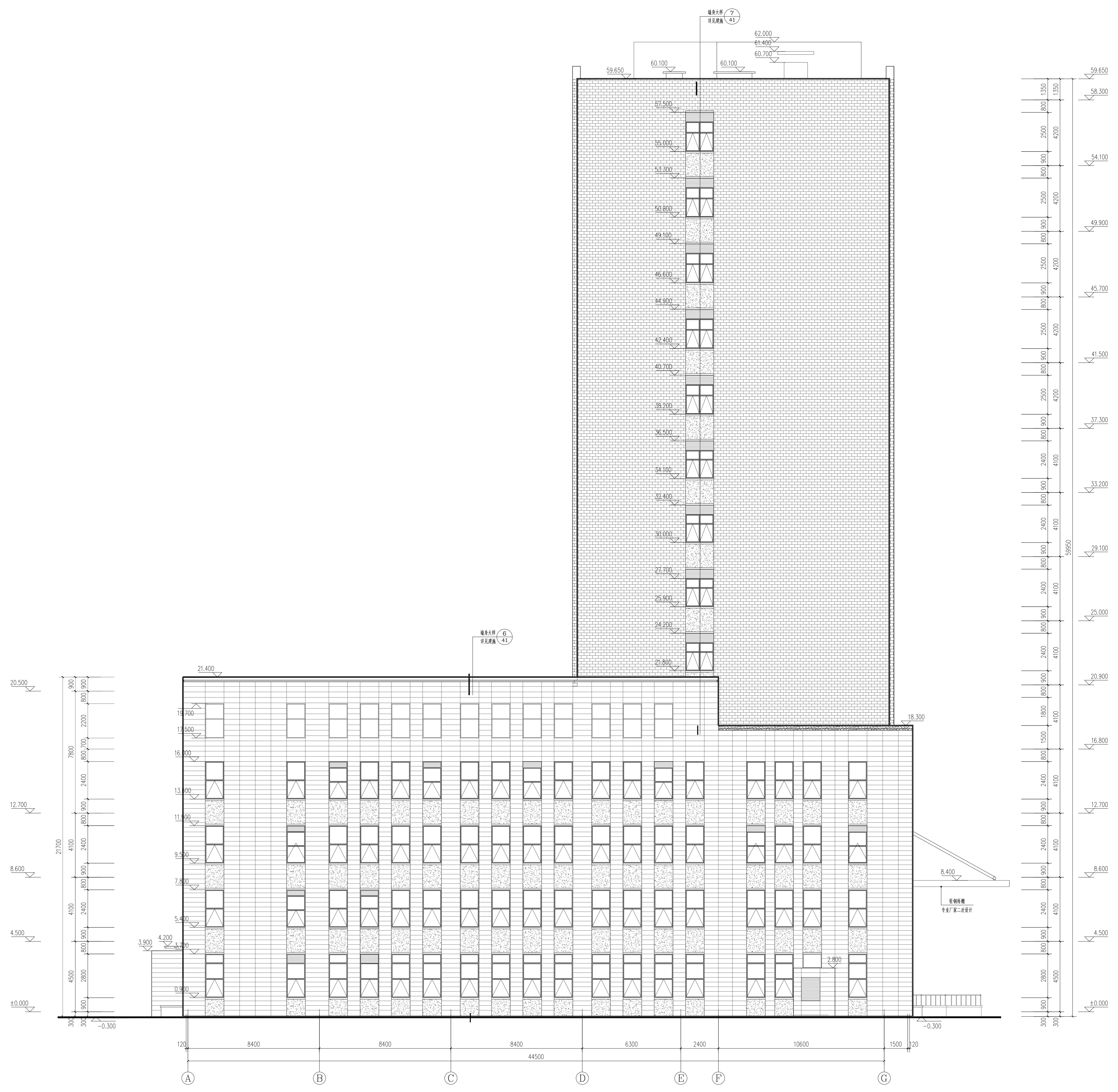
①~⑥立面图 1:100
